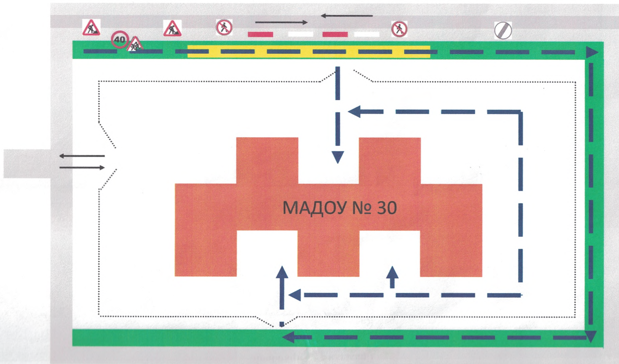
План-схема пути движения транспортных средств и детей при проведении дорожных ремонтно-строительных работ вблизи МАДОУ № 30
